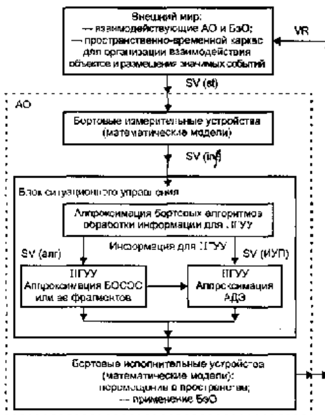
Рисунок 1 – Облик ИММ-ПГУУ(R)/
