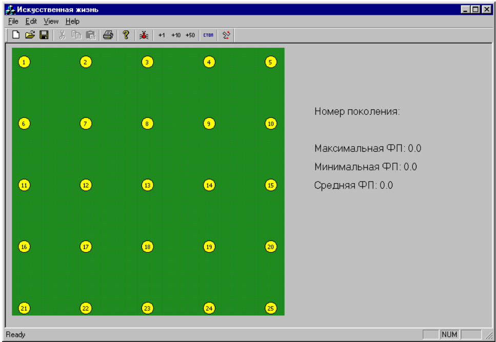
Рисунок 2 – Пространство поиска.
